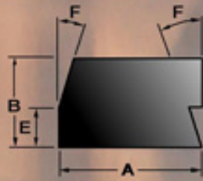
Profil-Nr. 14717 CCNB
