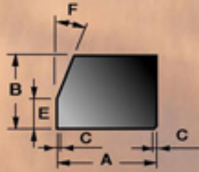
Profil-Nr. 13946 CCNB
