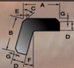
Profil-Nr. 13200 CCNB
