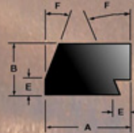
Profil-Nr. 15691 CCNB
