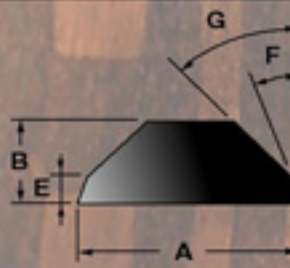
Profil-Nr. 15825 CCNB
