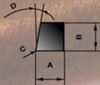
Zincir Profili
